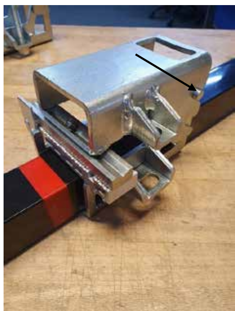
Stahlbefestigungsklemme (neu) Version Position-1 (Pfeil) / Level +1 = mit einem Distanzstück (Spacer) => +15 mm Version position one (see arrow) / Level +1 = with one spacer => +15 mm
